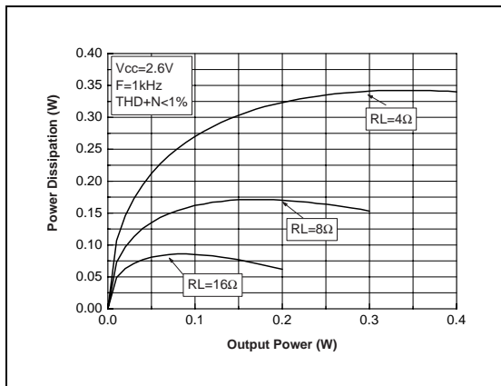
Fig. 19 : Power Dissipation vs Pout
