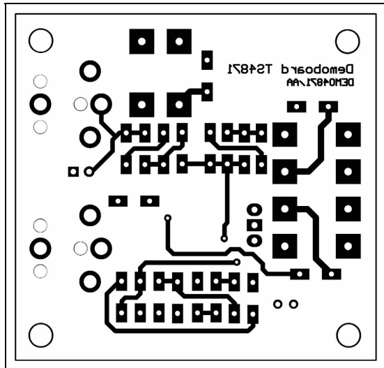
Fig. 84 : SO8 & MiniSO8 Demoboard Bottom Solder Layer
