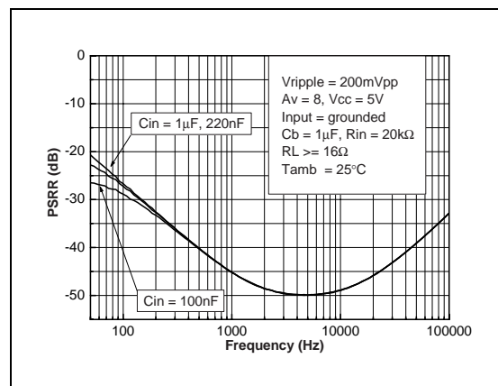
Fig. 94: PSRR vs Input Capacitor
