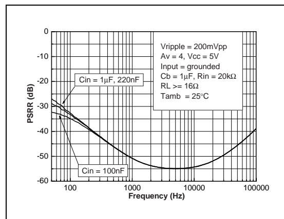
Fig. 73: PSRR vs Input Capacitor
