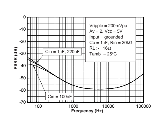
Fig. 51: PSRR vs Input Capacitor
