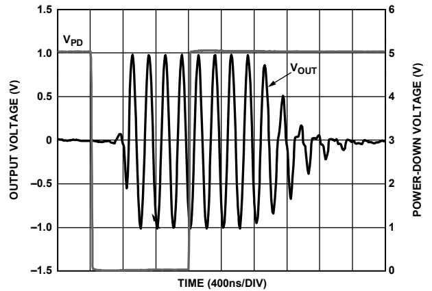
Figure 27. Enable/Power-Down Time
