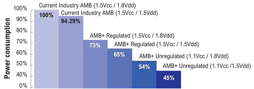
Type of AMB technology Ultra low power FB-DIMM enabled by IDT AMB+
