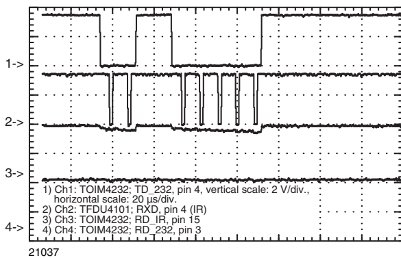
Fig. 11 - Echo-Suppression
