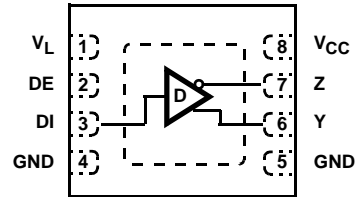
ISL3296E, ISL3297E, ISL3298E (8 LD TDFN) TOP VIEW
