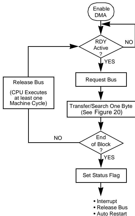
Figure 21. Byte Mode
