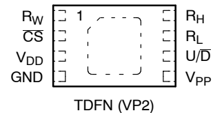
TDFN (VP2)
