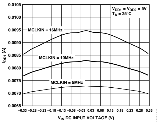
Figure 14. I DD1 vs. V IN DC Input Voltage
