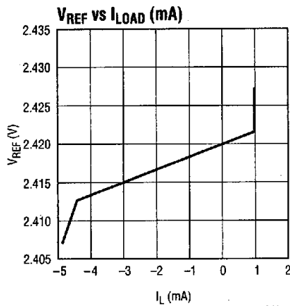
LT1272-TPC06
