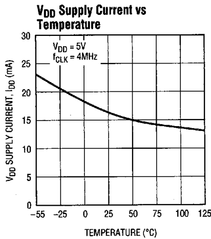
LT1272-TPC03
