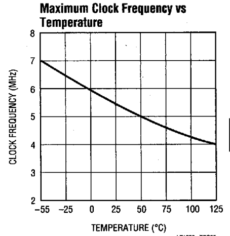
LT1272-TPC05
