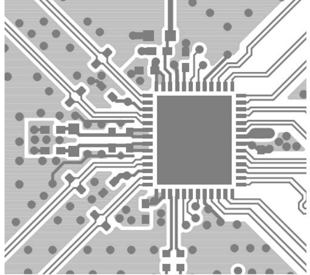
Top Side
