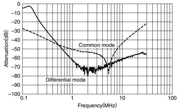
RSEL-2003W/A
