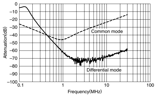
RSEL-2003WL/AL
