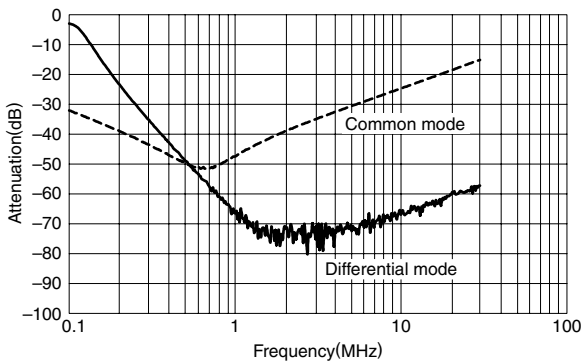
RSEL-2002WL/AL
