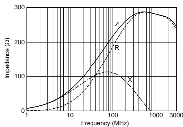
BLM15EG221SN1
