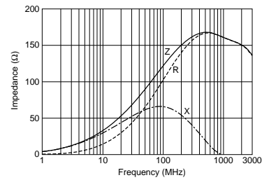
BLM15EG121SN1
