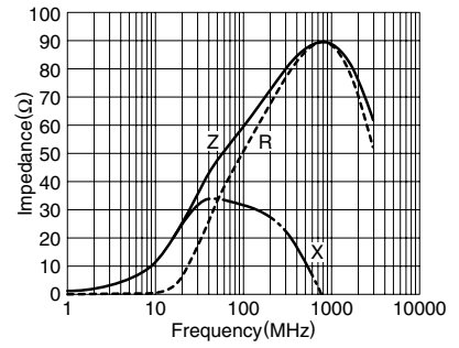
MPZ1005S600C
