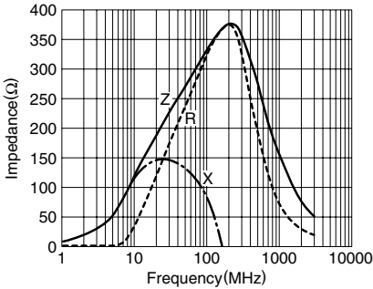
MPZ2012S331A
