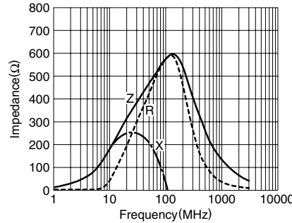
MPZ2012S601A
