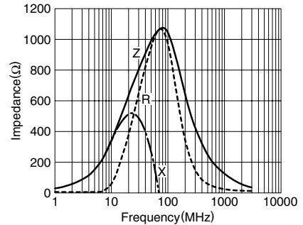
MPZ2012S102A
