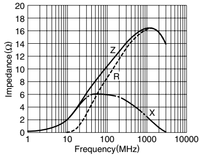
MPZ1005S121C
