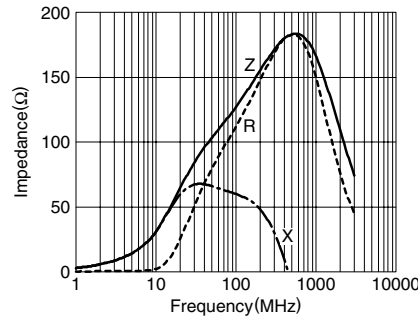
MPZ1608S331A
