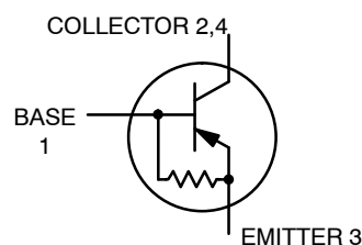
SOT-223 CASE 318E STYLE 1
