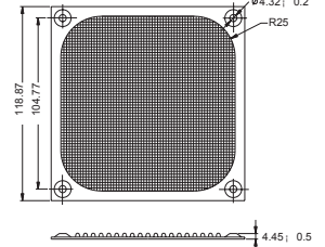
FM 12 For 120mm Fan
