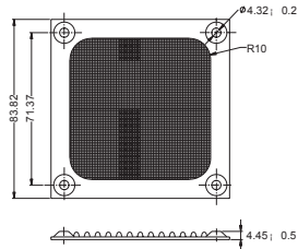
FM 08 For 80mm Fan
