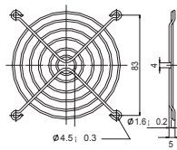
FG-09 For 92mm Fan
