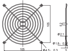
FG-12 For 120mm Fan
