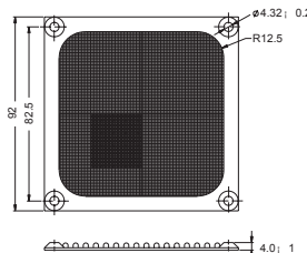
FM 09 For 92mm Fan
