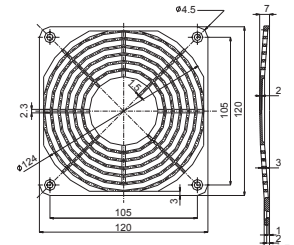
PB-12 For 120mm Fan
