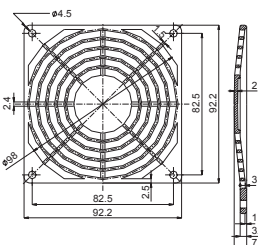
PB-09 For 92mm Fan
