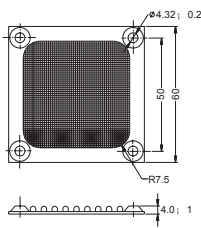
FM 06 For 60mm Fan
