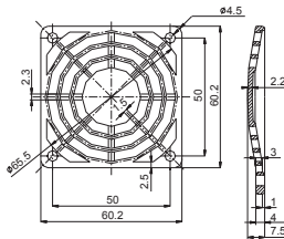
PB-06 For 60mm Fan
