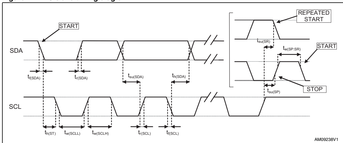
Figure 4. I 2 C slave timing diagram (d)
