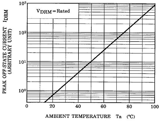
NORMALIZED I_{DRM} - T_a
