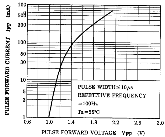
I_{FP} - V_{FP}
