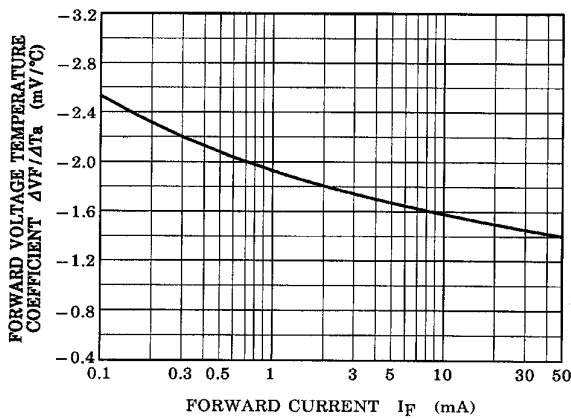
\Delta V_F / \Delta T_a - I_F
