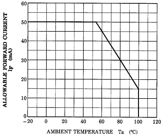
I_F - T_a
