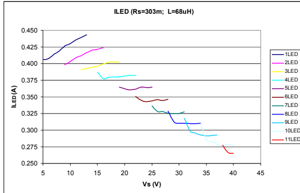
ILD4035_ILED_303m_68u.vsd
