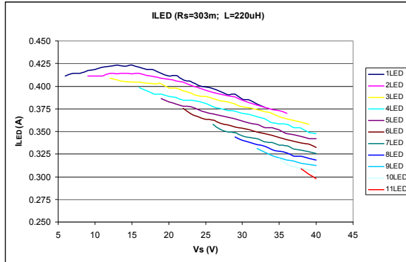
ILD4035_ILED_303m_220u.vsd
