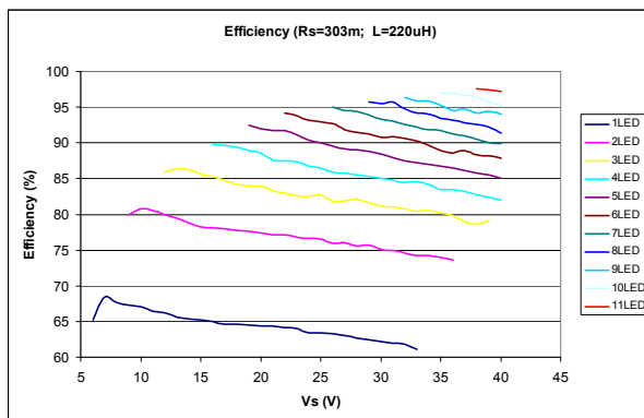
ILD4035_Efficiency_303m_220u.vsd
