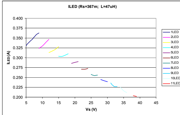
ILD4035_ILED_367m_47u.vsd
