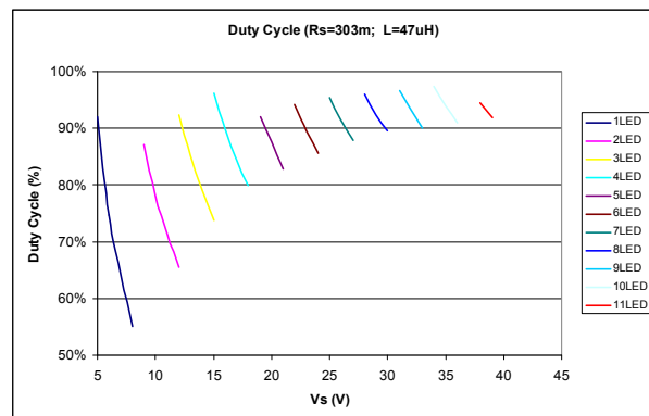
ILD4035_Duty_Cycle_303m_47u.vsd
