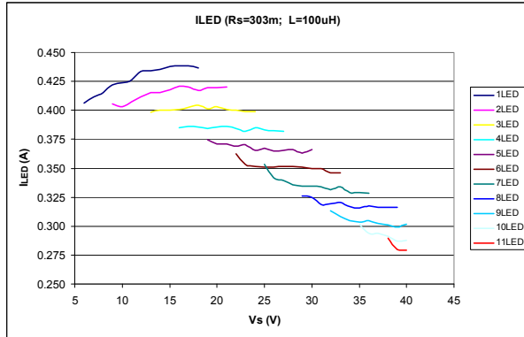
ILD4035_ILED_303m_100u.vsd
