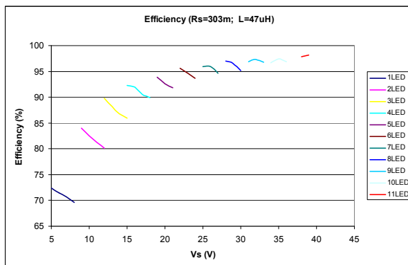
ILD4035_Efficiency_303m_47u.vsd
