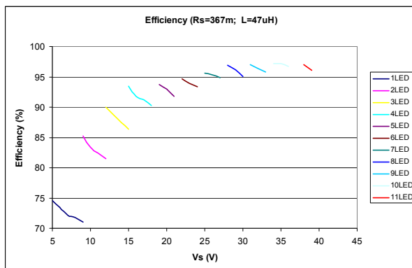
ILD4035_Efficiency_367m_47u.vsd
