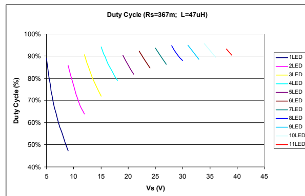
ILD4035_Duty_Cycle_367m_47u.vsd
