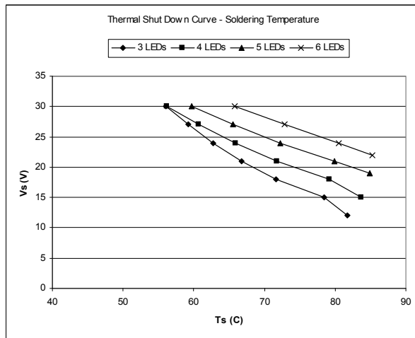
ILD4035_TSD_over_Ts.vsd
