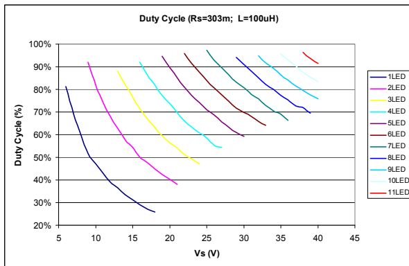
ILD4035_Duty_Cycle_303m_100u.vsd
