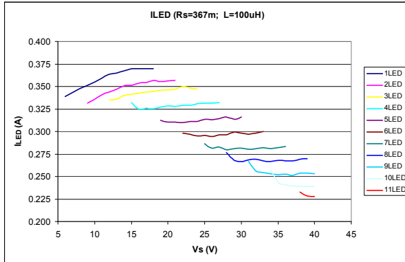
ILD4035_ILED_367m_100u.vsd
