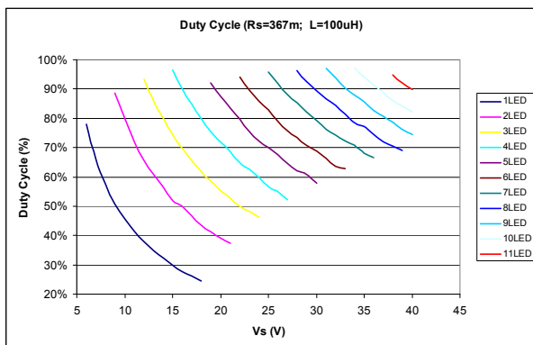
ILD4035_Duty_Cycle_367m_100u.vsd
