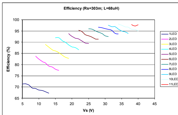
ILD4035_Efficiency_303m_68u.vsd
