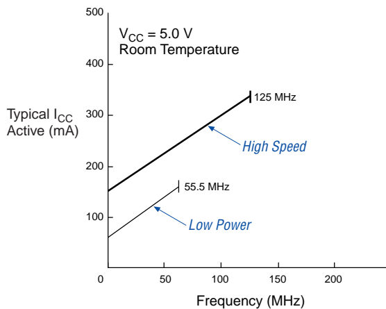
EPM7128E
