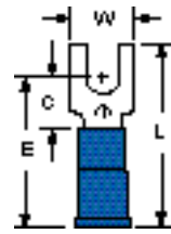
MVU14-8FB Stud Size: 8 Wire Range: 16-14
