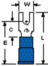
MVU14-4FB/S Stud Size: 4 Wire Range: 16-14
