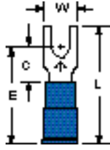
MVU14-6FB/S Stud Size: 6 Wire Range: 16-14
