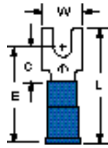
MVU14-6FB Stud Size: 6 Wire Range: 16-14
