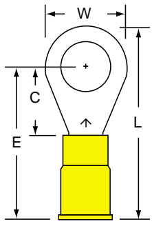
MVU10-516R/S Stud Size: 5/16 Wire Range: 12-10
