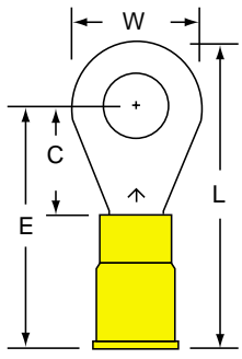
MVU10-14R/S Stud Size: 1/4 Wire Range: 12-10
