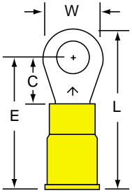
MVU10-10R Stud Size: 10 Wire Range: 12-10
