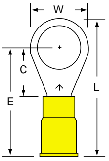
MVU10-38R/S Stud Size: 3/8 Wire Range: 12-10
