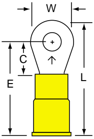
MVU10-8R Stud Size: 8 Wire Range: 12-10
