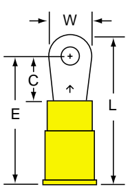
MVU10-4R/S Stud Size: 4 Wire Range: 12-10
