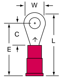
MVU18-8R/L Stud Size: 8 Wire Range: 22-18
