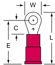
MVU18-6R/S Stud Size: 6 Wire Range: 22-18
