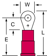
MVU18-4R/S Stud Size: 4 Wire Range: 22-18
