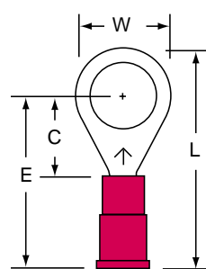
MVU18-516R/S Stud Size: 5/16 Wire Range: 22-18
