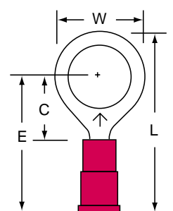
MVU18-38R Stud Size: 3/8 Wire Range: 22-18
