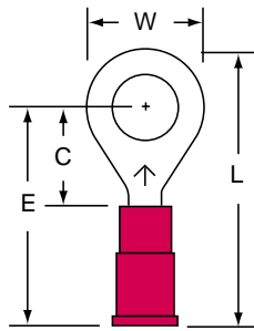
MVU18-14R/S Stud Size: 1/4 Wire Range: 22-18
