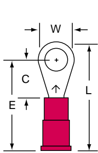
MVU18-10R/L Stud Size: 10 Wire Range: 22-18
