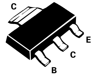
SOT223
