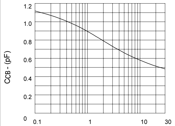
CCB v VCB
