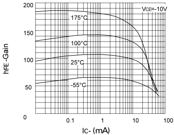
hFE v IC
