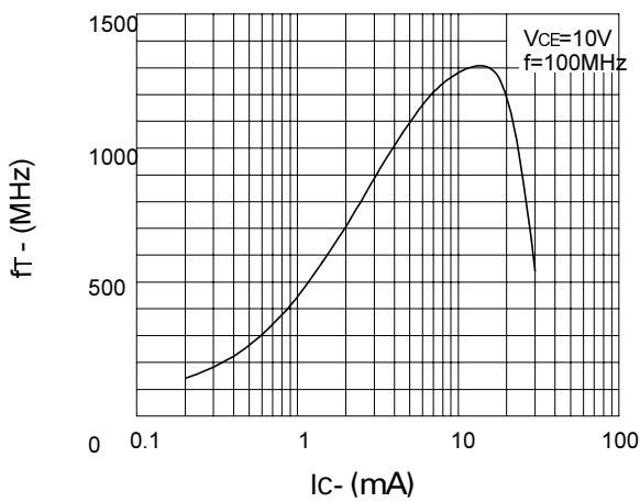
fT v IC
