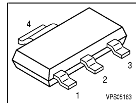
PG-SOT-223
