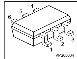
PG-SOT-363
