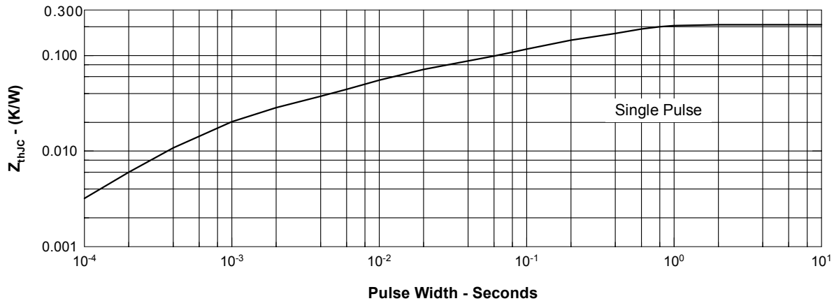
Fig. 10. Thermal Impedance
