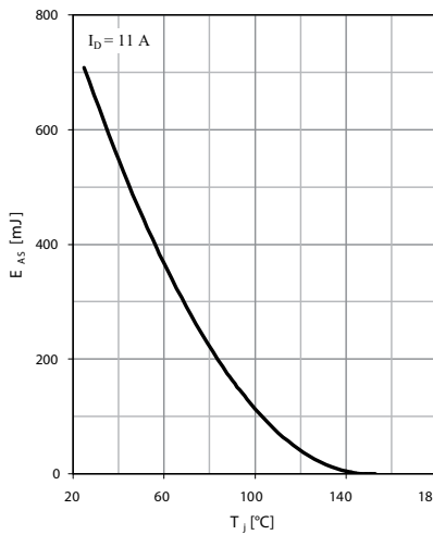
Fig. 10 Avalanche energy
