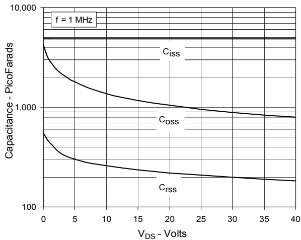
Fig. 11. Capacitance
