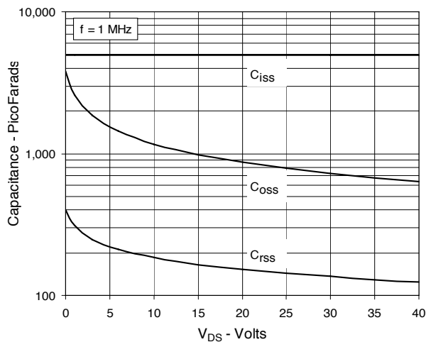
Fig. 11. Capacitance
