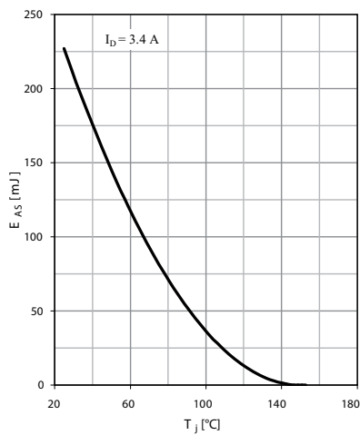
Fig. 10 Avalanche energy
