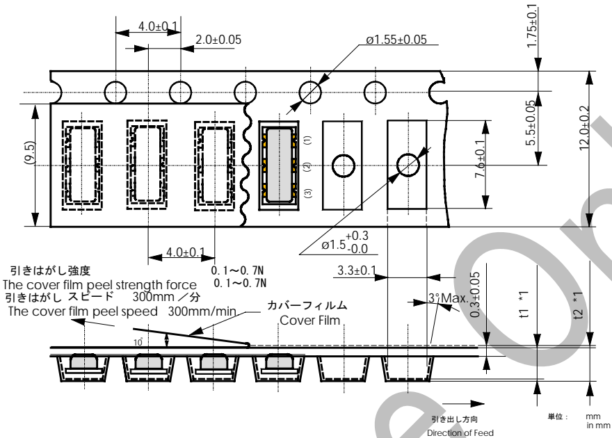
第3図 プラスチックテープの外形寸法図 Figure 3. Dimensions of Plastic Tape (CSTCC8M00G53-R0)
