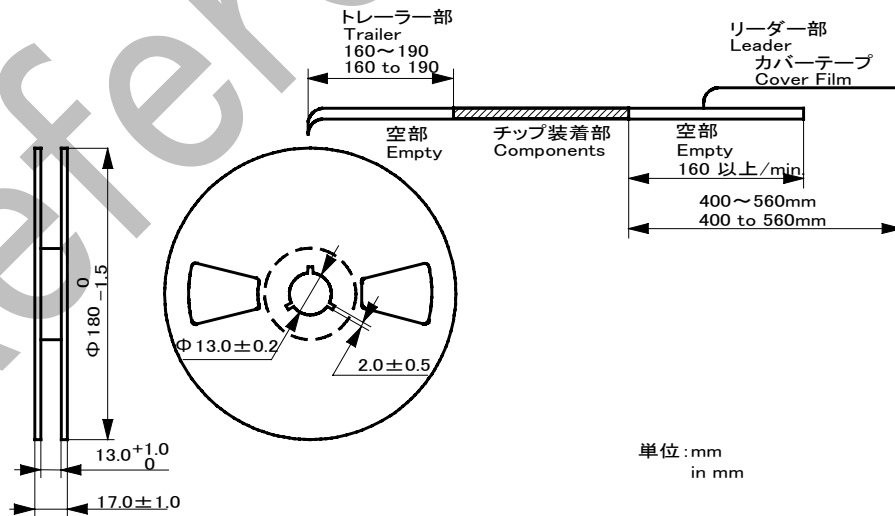
第4図 プラスチックリールの外形寸法図 Figure 4. Dimensions of Plastic Reel (CSTCC8M00G53-R0)
