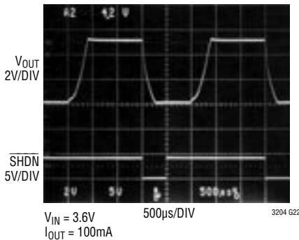
VOUT Soft-Start
