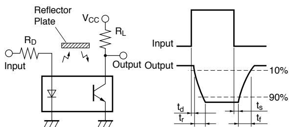
Fig.9 応答時間の測定回路
