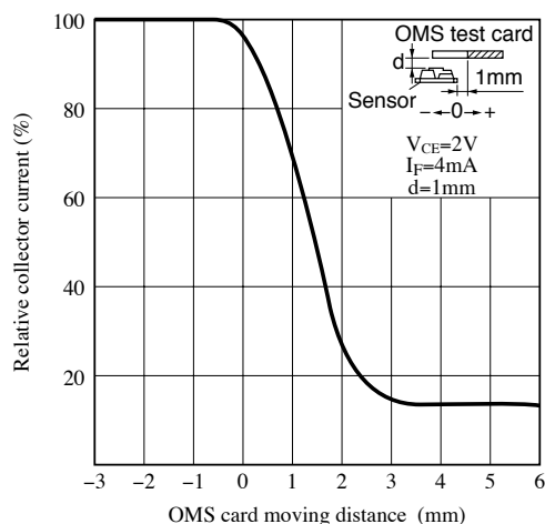
Fig.12 検出位置特性 (1)
