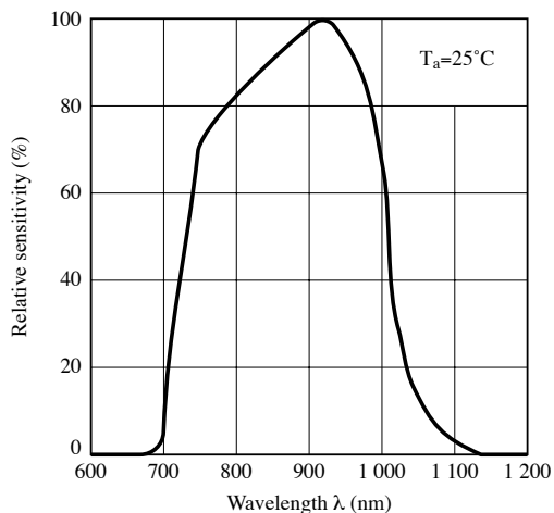
Fig.11 分光感度特性 (受光側)
