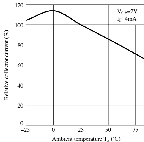
Fig.6 相对光電流—周囲温度特性
