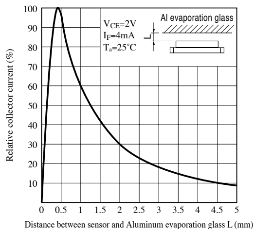
Fig.12 検出位置特性 (1)
