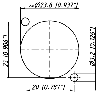
Frontplattenausschnitt (Frontseite) Panel cut out (front side)
