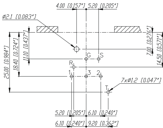
Print-Bohrplan (Bestückungsseite) PCB-Layout (component side)
