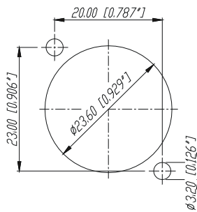
Frontplattenausschnitt (Frontseite) Panel cut out (front side)
