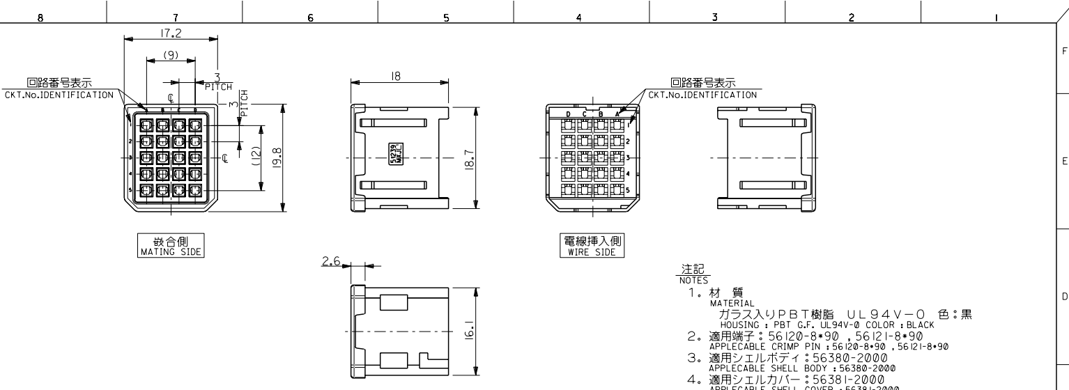
<誤嵌合防止キー(極性)タイプ> <POLARITY KEY TYPE>
