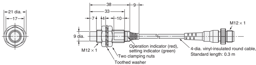
Fig. 32: E2E-X7D1-M1GJ E2E-X7D1-M1J-T
