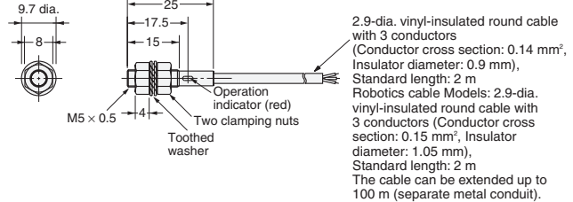
Fig. 4: E2E-X1
