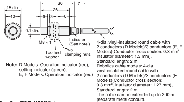
Fig. 8: E2E-X2MY
