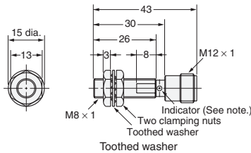
Fig. 18: E2E-X2D□-M1(G) E2E-X1R5E□-M1/F□-M1
