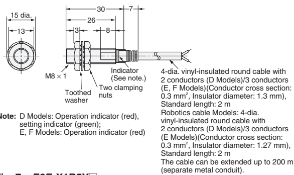
Fig. 7: E2E-X1R5Y
