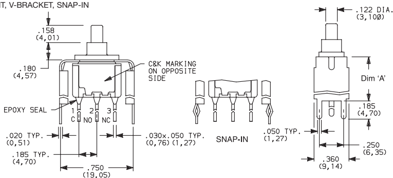
8121SD3_GE SPDT
