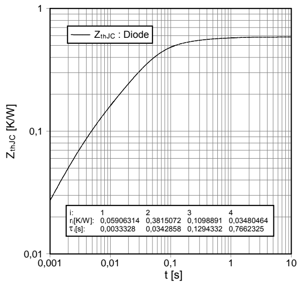
Transienter Wärmewiderstand Diode-Wechsler. transient thermal impedance diode-inverter
