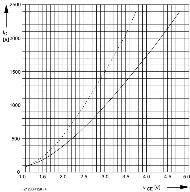
Bild/Fig. 1 Kollektor-Emitter-Spannung im Sättigungsbereich (typisch) Collector-emitter-voltage in saturation region (typical) V_{GE} = 15\text{V} --- T_{vj} = 25^\circ\text{C} — T_{vj} = 125^\circ\text{C}
