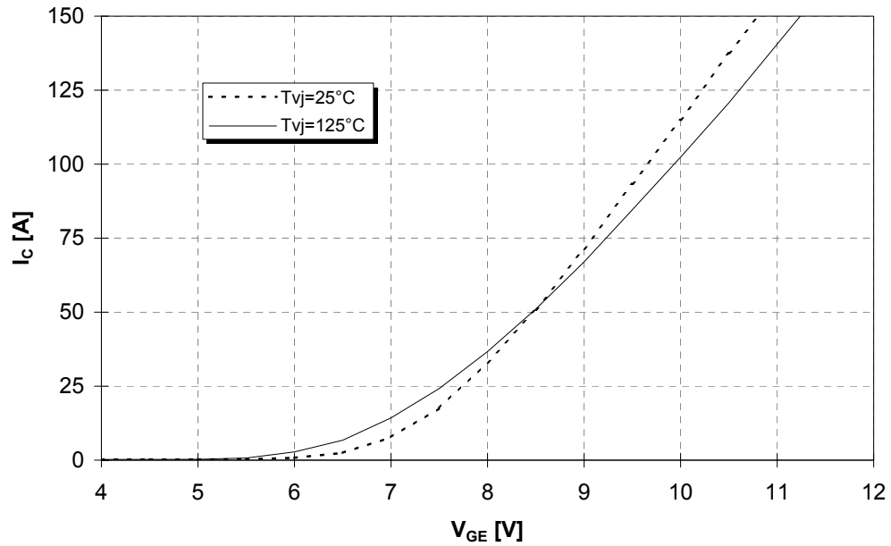
Übertragungscharakteristik (typisch) transfer characteristic (typical)
