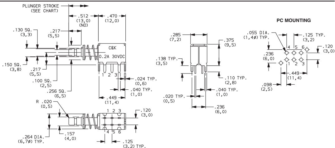
PN21LASA03QE DPDT
