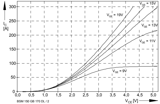
Bild / Fig. 2 Ausgangskennlinienfeld (typisch) / Output characteristic (typical) I_C = f(V_{CE}) T_{vj} = 125°C
