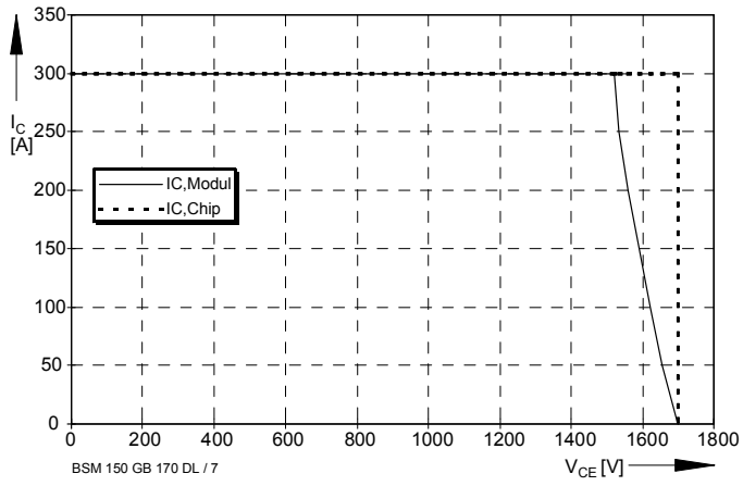
Bild / Fig. 7 Sicherer Arbeitsbereich (RBSOA) / Reverse bias safe operation area (RBSOA) R_{\theta} = 10\Omega , T_{vj} = 125^{\circ}\text{C}
