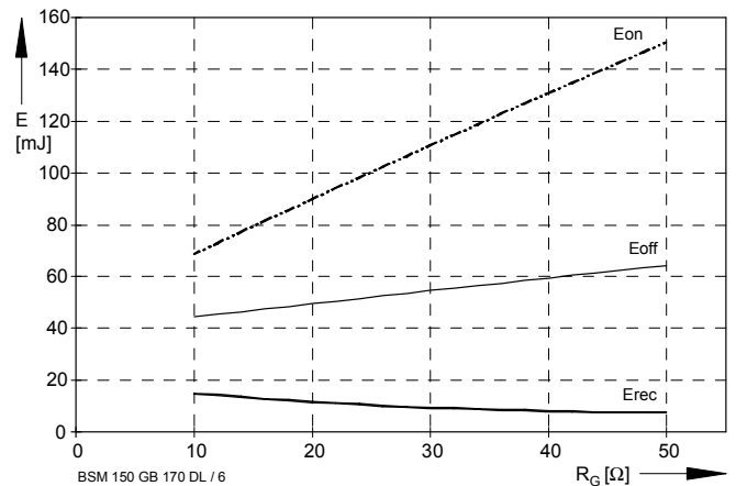
Bild / Fig. 6 Schaltverluste (typisch) / Switching losses (typical) E_{on} = f(R_G) , E_{off} = f(R_G) , E_{rec} = f(R_G) I_C = 150A , V_{CE} = 900V , T_j = 125°C
