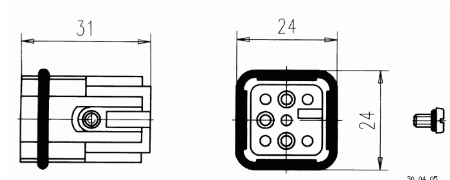
Maßzeichnung Dimensions in mm (Inch)
