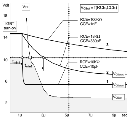
Fig.6 V_{CEsat} waveform with parameters R_{CE} , C_{CE}
