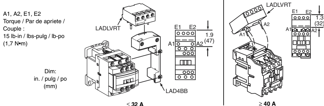
Figure / Figura / Figure 1 : Contactors / Contactores / Contacteurs
