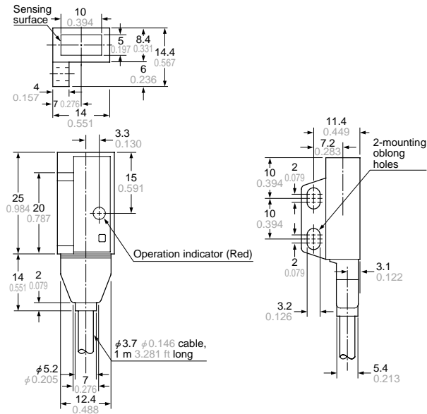
PM2-LL10-C1 PM2-LL10B-C1 Sensor
