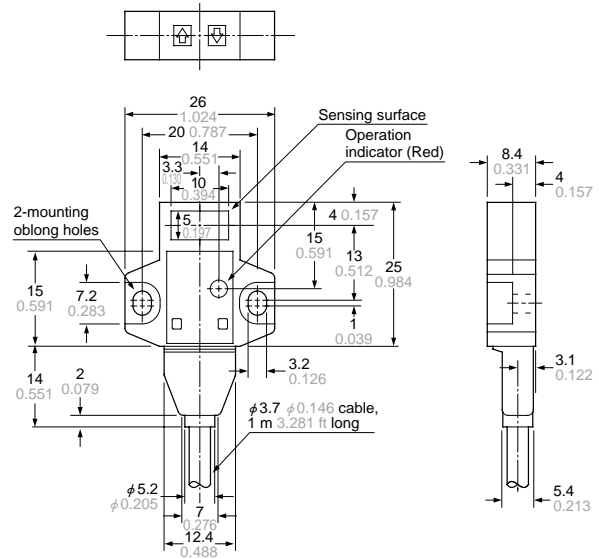
PM2-LF10-C1 PM2-LF10B-C1 Sensor
